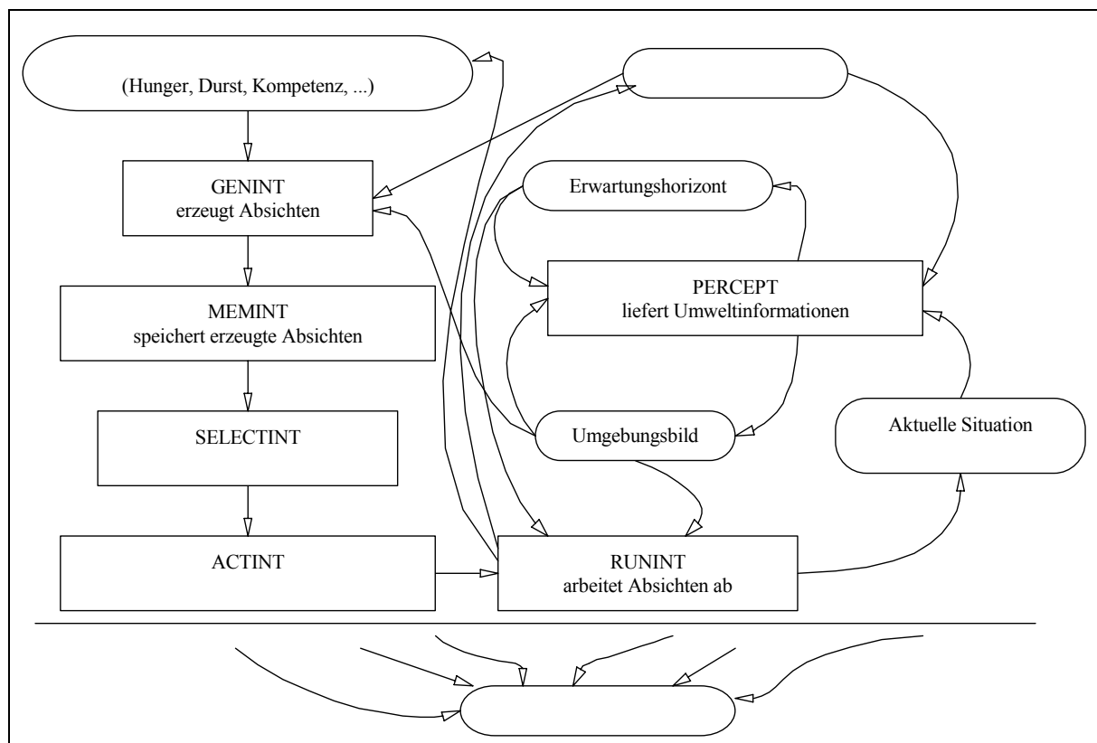
Abbildung 2: Übersicht über die PSI-Prozesse.
